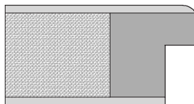
KŘÍDLO S POLODRÁŽKOU zaoblená hrana křídla hrana R6
