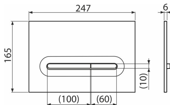
Ovládací tlačítko pro předstěnové instalační systémy, bílá mat
