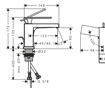
HANSGROHE Baterie umyvadlová stojánková páková Tecturis E 80 CoolStart bez odtokové soupravy, chrom
