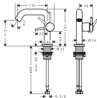
HANSGROHE TECTURIS S 110 Fine umyvadlová stojánková baterie, s odtokovou soupravou, CoolStart, EciSmart+, chrom
