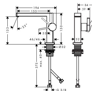
HANSGROHE TECTURIS E 110 Fine umyvadlová stojánková baterie, s odtokovou soupravou, CoolStart, EciSmart+, chrom
