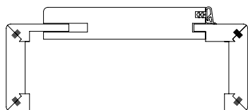
OBLOŽKOVÁ ZÁRUBEŇ zaoblená R3 – 60 mm
